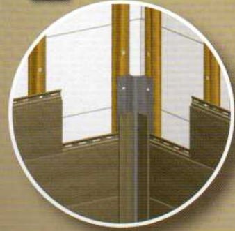
Wykończenie narożnika wewnętrznego
