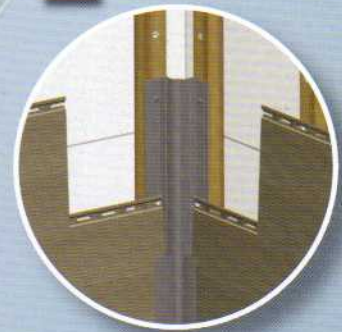
Naróżnik wewnętrzny profil 2
